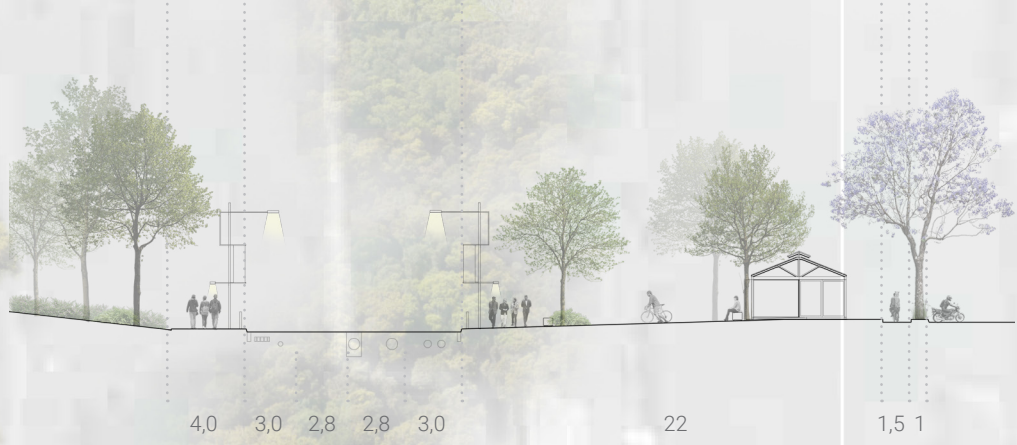
ampliação 1 _ corte 1:400
