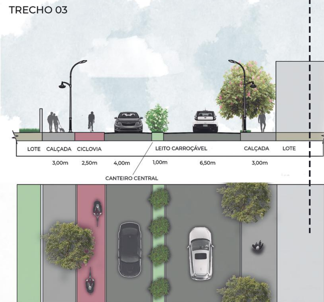
CORTE A VIA PROPOSTA EM PROJETO
