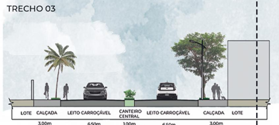
CORTE A VIA EM SITUAÇÃO ATUAL
